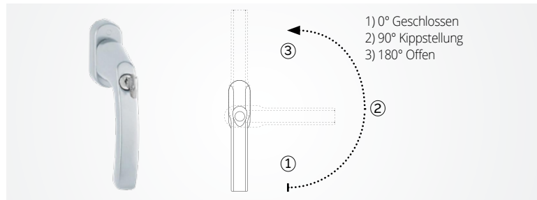
TBT BESCHLAG (TILT BEFORE TURN)
