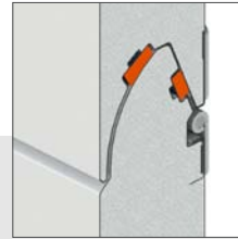
Paneel von 60 mm Stärke. U=0,9 \text{ [W/m}^2\text{K]}^*
