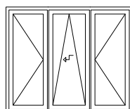
3-teiliges Element mit Schiebeflügel und zwei Drehflügeln
