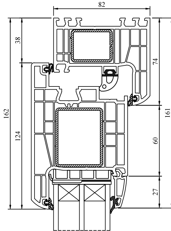
A - A
