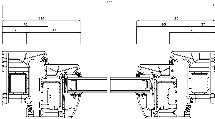
Schnitt S2(5:1)
