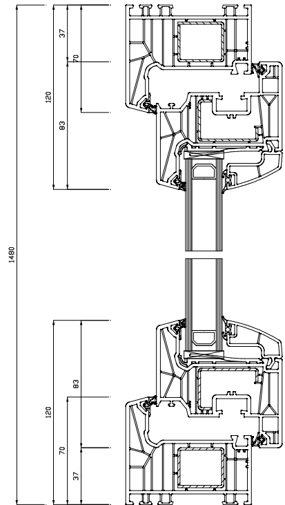
Schnitt S1(5:1)
