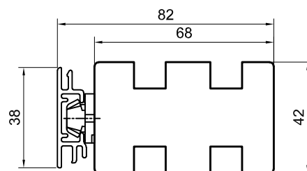
PRD 042 - poszerzenie 42mm PRD 042 - verbreiterung 42mm PRD 042 - Allargamento 42mm
