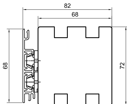
PRD 072 - poszerzenie 72mm PRD 072 - verbreiterung 72mm PRD 072 - Allargamento 72mm
