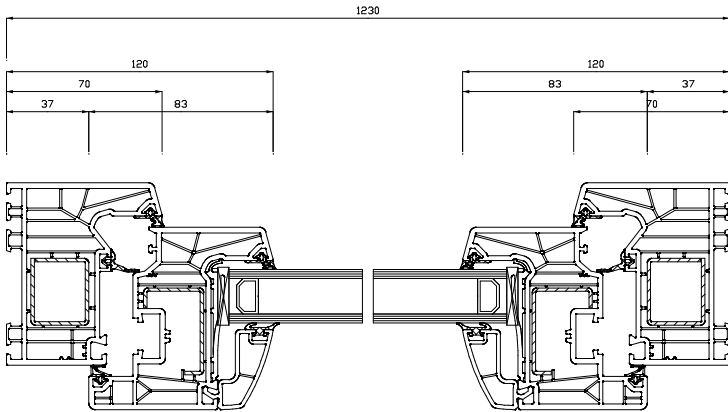
Schnitt S2(5:1)
