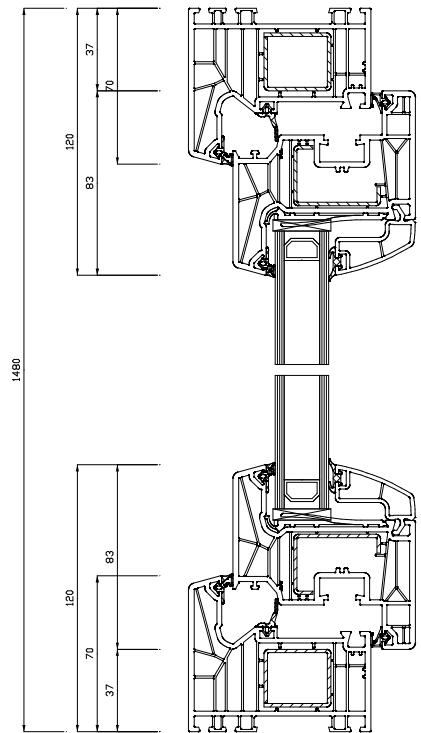
Schnitt S1(5:1)
