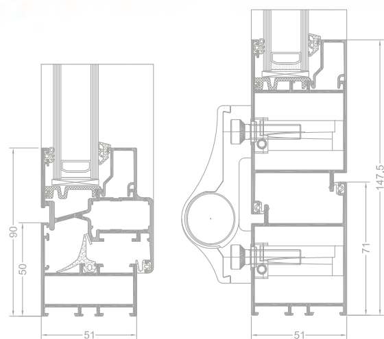
Querschnitt durch ein Fenster EL 010 + VL 820
