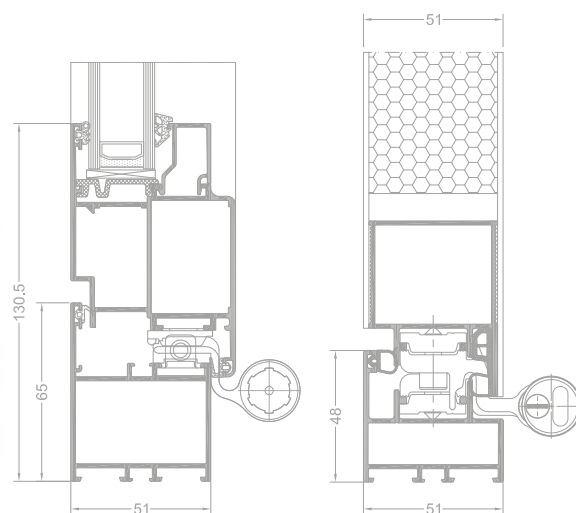
Querschnitt durch ein Fenster EL 011 + EL 022
