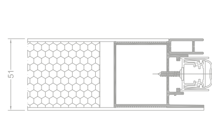
Querschnitt durch eine Paneeltür - Option mit absinkender Schwelle
